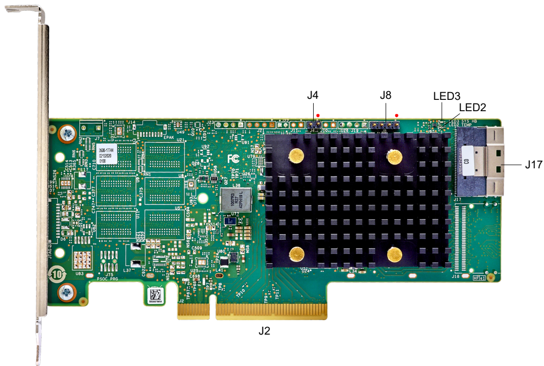
Figura 1: Diseño de tarjeta del HBA de 12 Gb ThinkSystem 440-8i SAS/SATA PCIe Gen4
