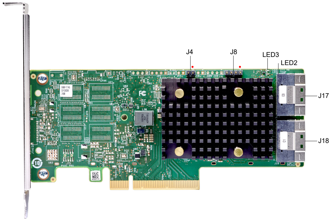
Figure 1 : Présentation du HBA ThinkSystem 440-16i SAS/SATA PCIe Gen4 12 Gbit
