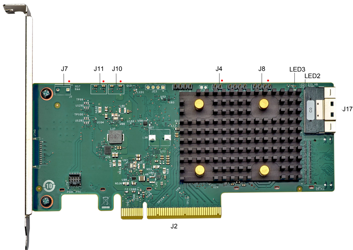
Figure 1 : Disposition de la carte pour l'adaptateur ThinkSystem RAID 540-8i PCIe Gen4 12 Gbit
