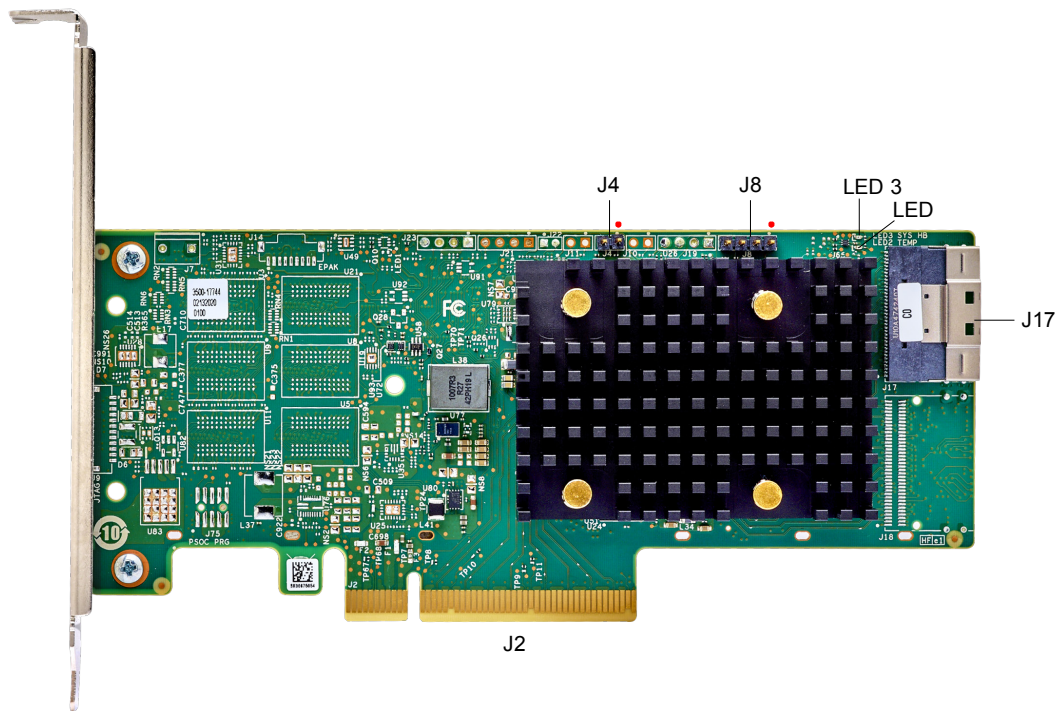
Figura 1 : layout della scheda di ThinkSystem 440-8i SAS/SATA PCIe Gen4 12 Gb HBA
