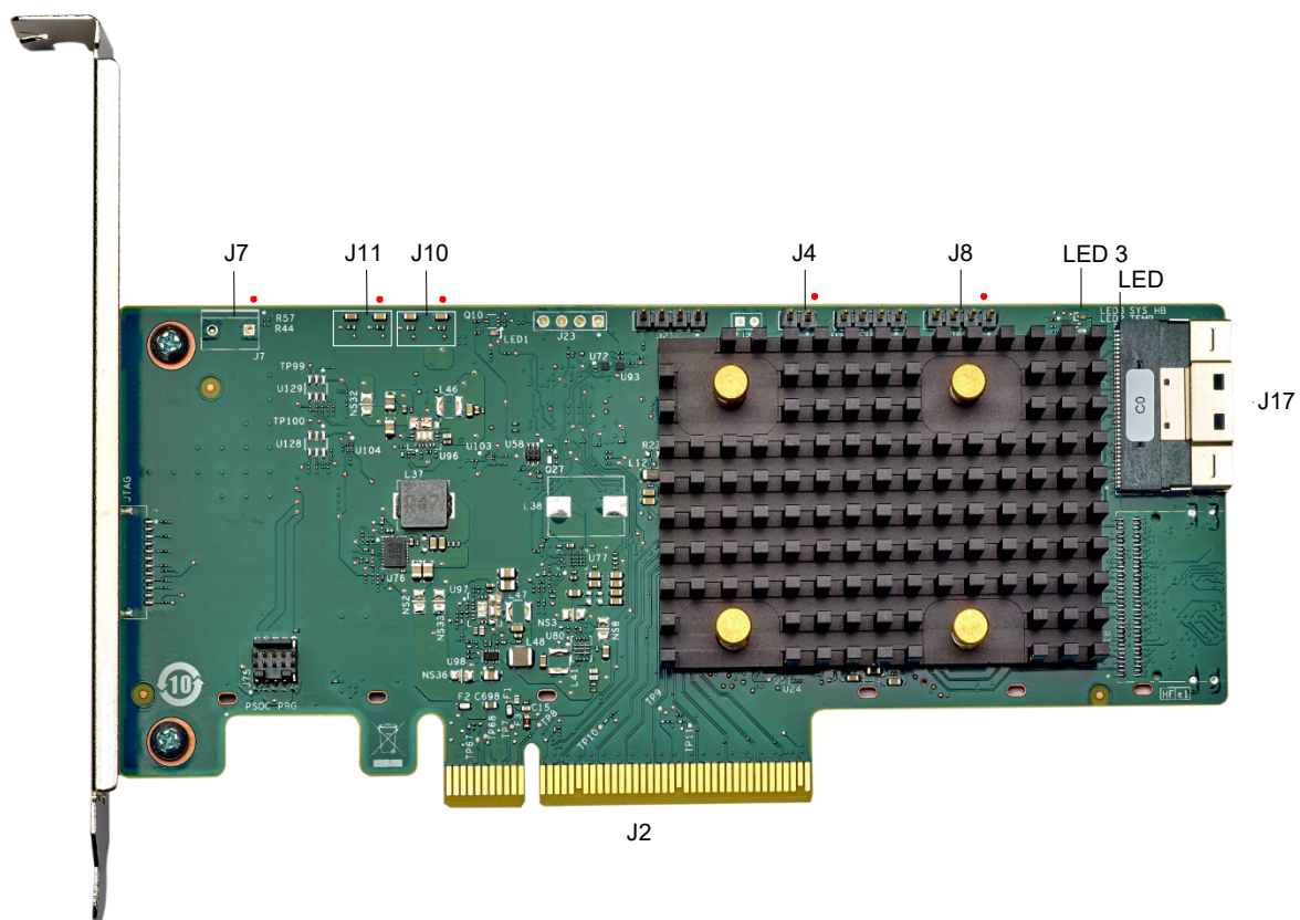
Figura 1: layout della scheda per l'adattatore ThinkSystem RAID 540-8i PCIe Gen4 12 Gb
