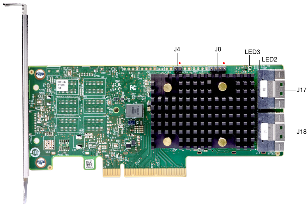
図 1: ThinkSystem 440-16i SAS/SATA PCIe Gen4 12Gb HBA のカード・レイアウト
