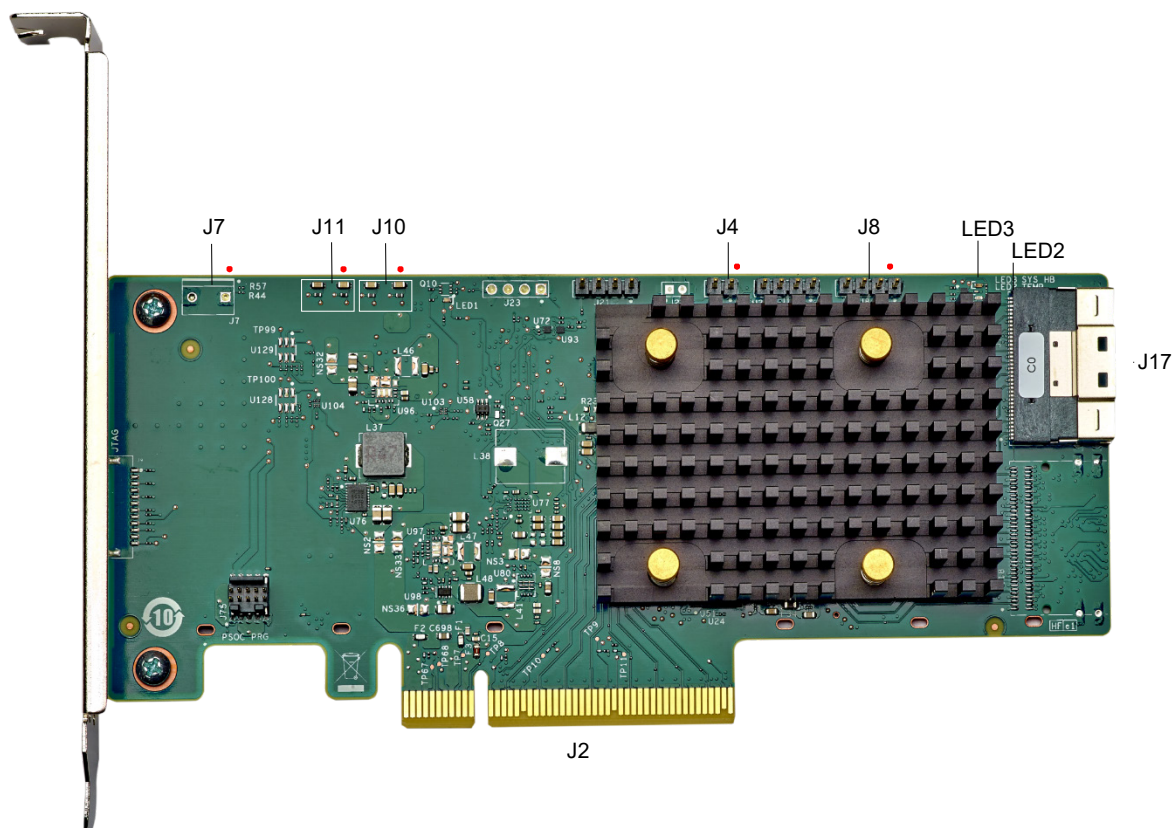
図 1: ThinkSystem RAID 540-8i PCIe Gen4 12Gb アダプターのカードのレイアウト
