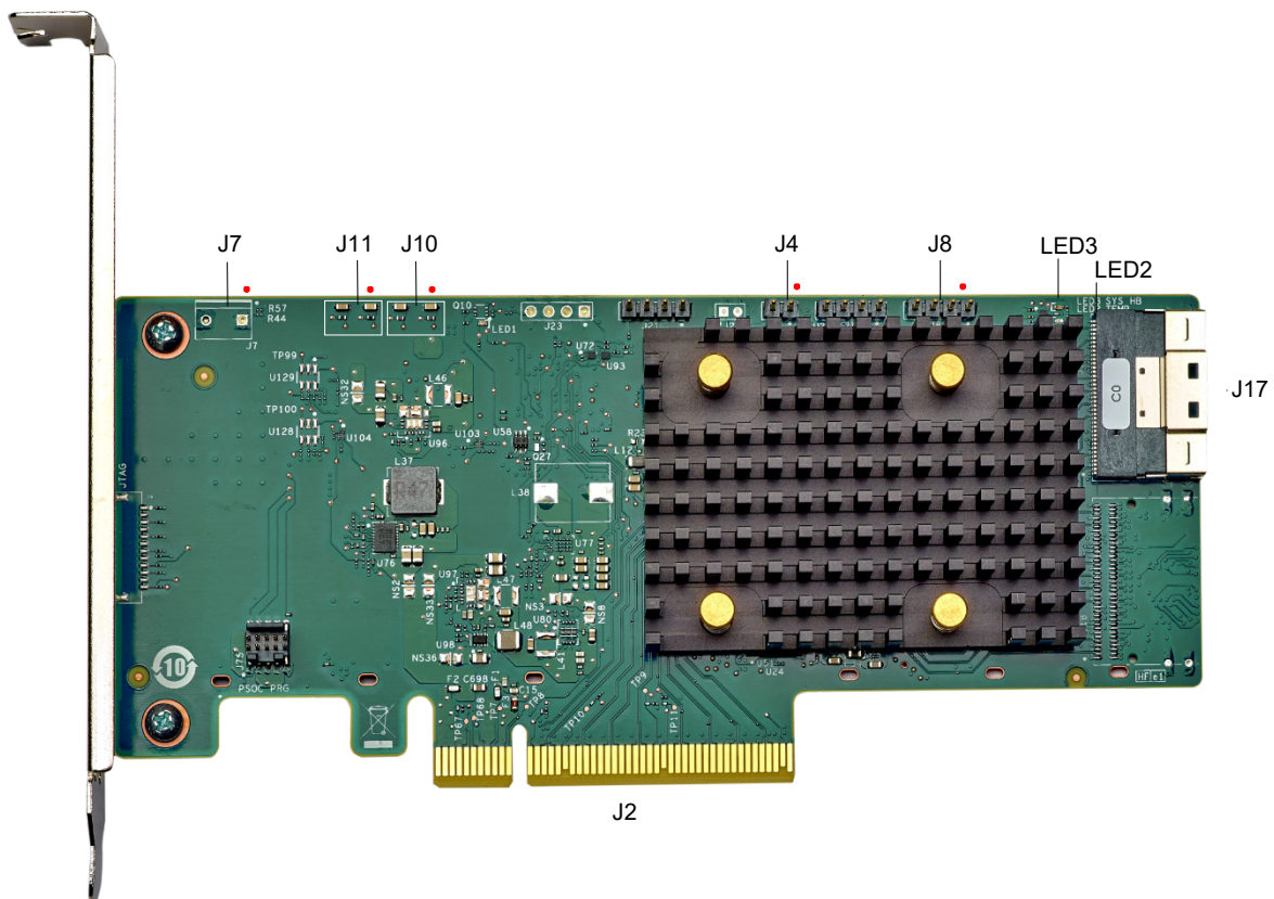
그림 1: ThinkSystem RAID 540-8i PCIe Gen4 12Gb 어댑터의 카드 레이아웃
