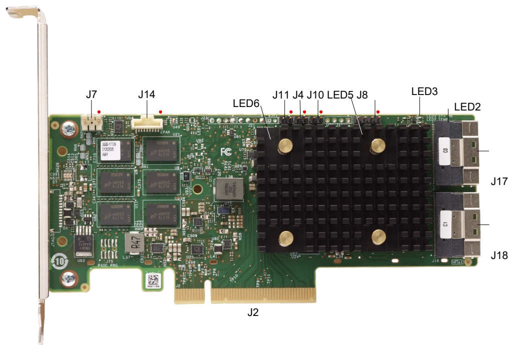
그림 1: ThinkSystem RAID 940-16i 4GB 플래시 PCIe Gen4 어댑터의 카드 레이아웃
