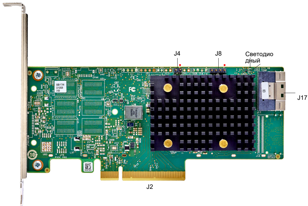
Рисунок 1. Компоновка плат адаптера ThinkSystem HBA 440-8i SAS/SATA PCIe Gen4 12 Гбит/с
