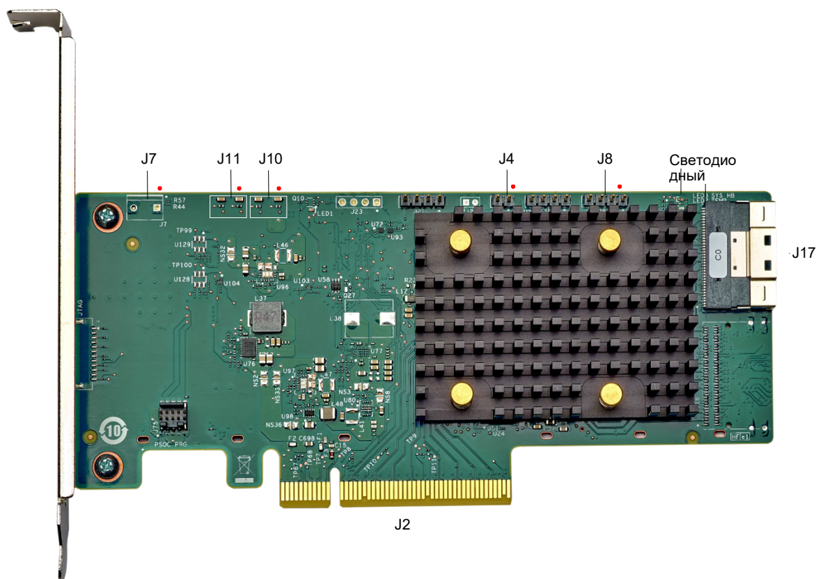
Рисунок 1. Компоновка плат адаптера ThinkSystem RAID 540-8i PCIe Gen4 12 Гбит/с
