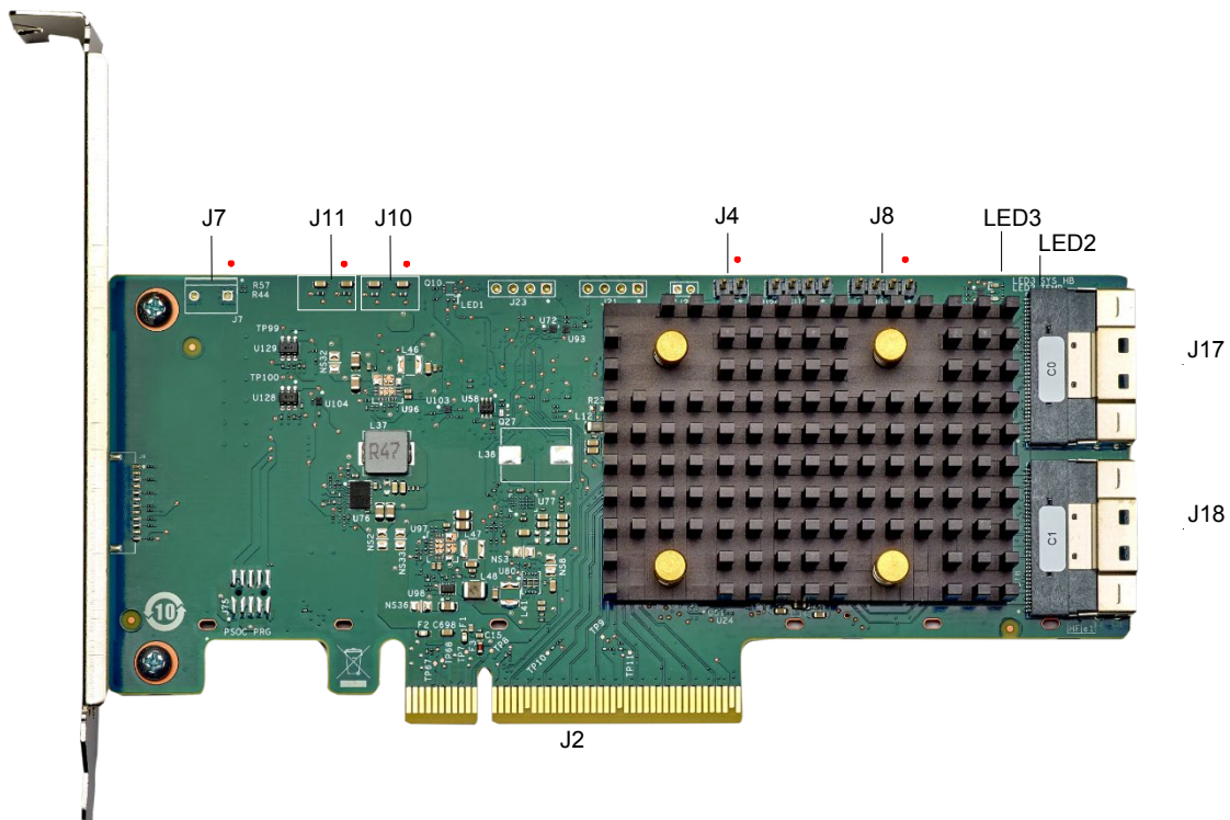
ภาพประกอบ 1: อะแดปเตอร์ RAID 540-16i PCIe Gen4 12Gb ของ ThinkSystem
