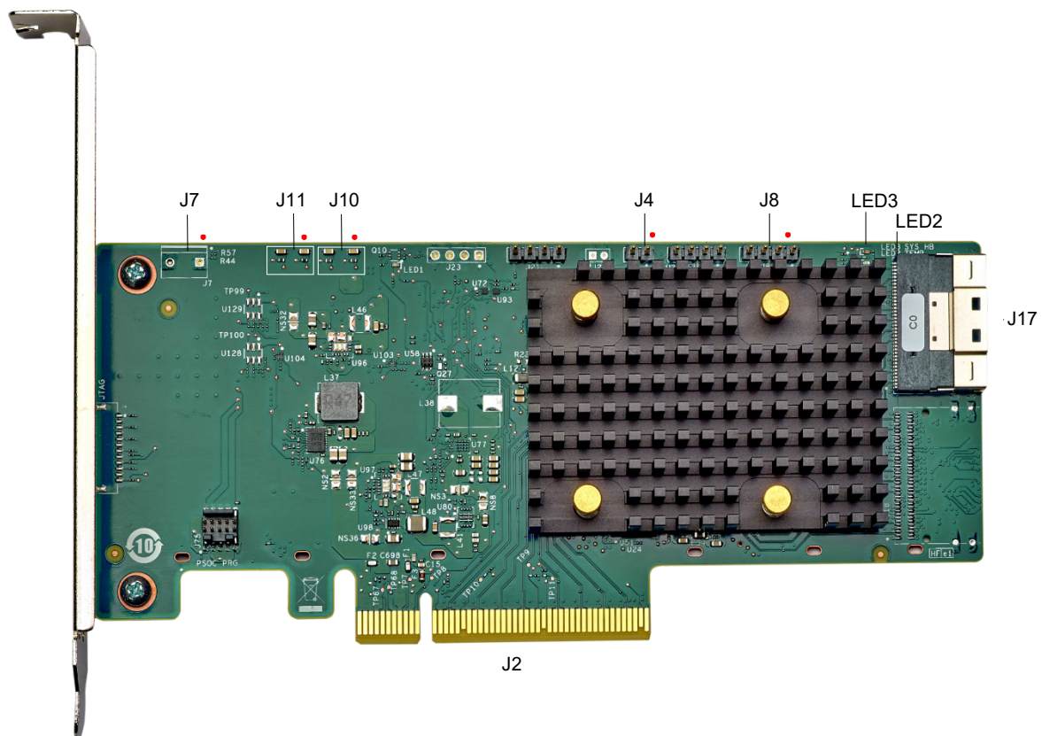
圖 1：ThinkSystem RAID 540-8i PCIe Gen4 12Gb 配接卡的卡片佈置
